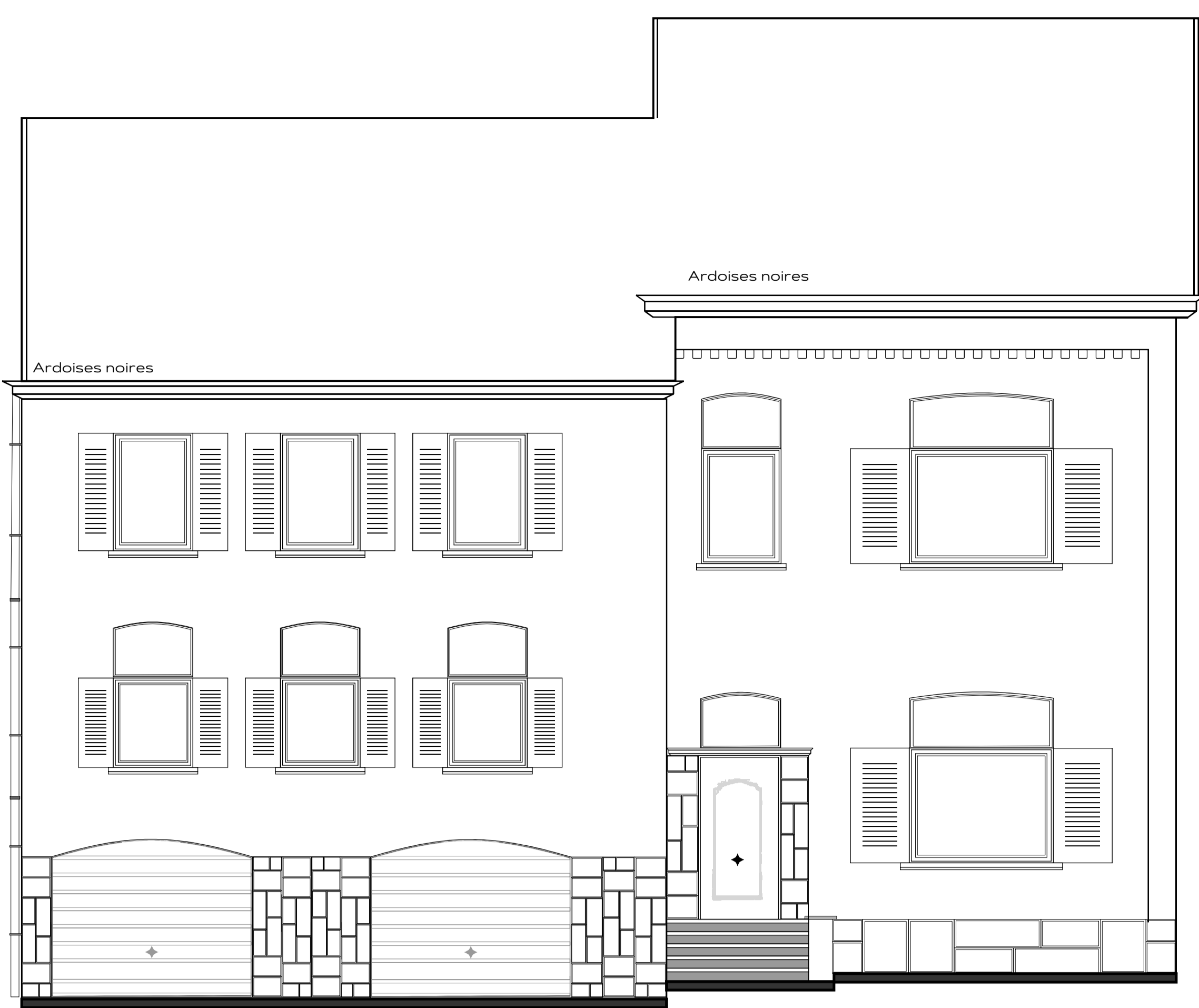
FACADE PRINCIPALE (à rue) Chaussée de Tirlemont-Charleroi
