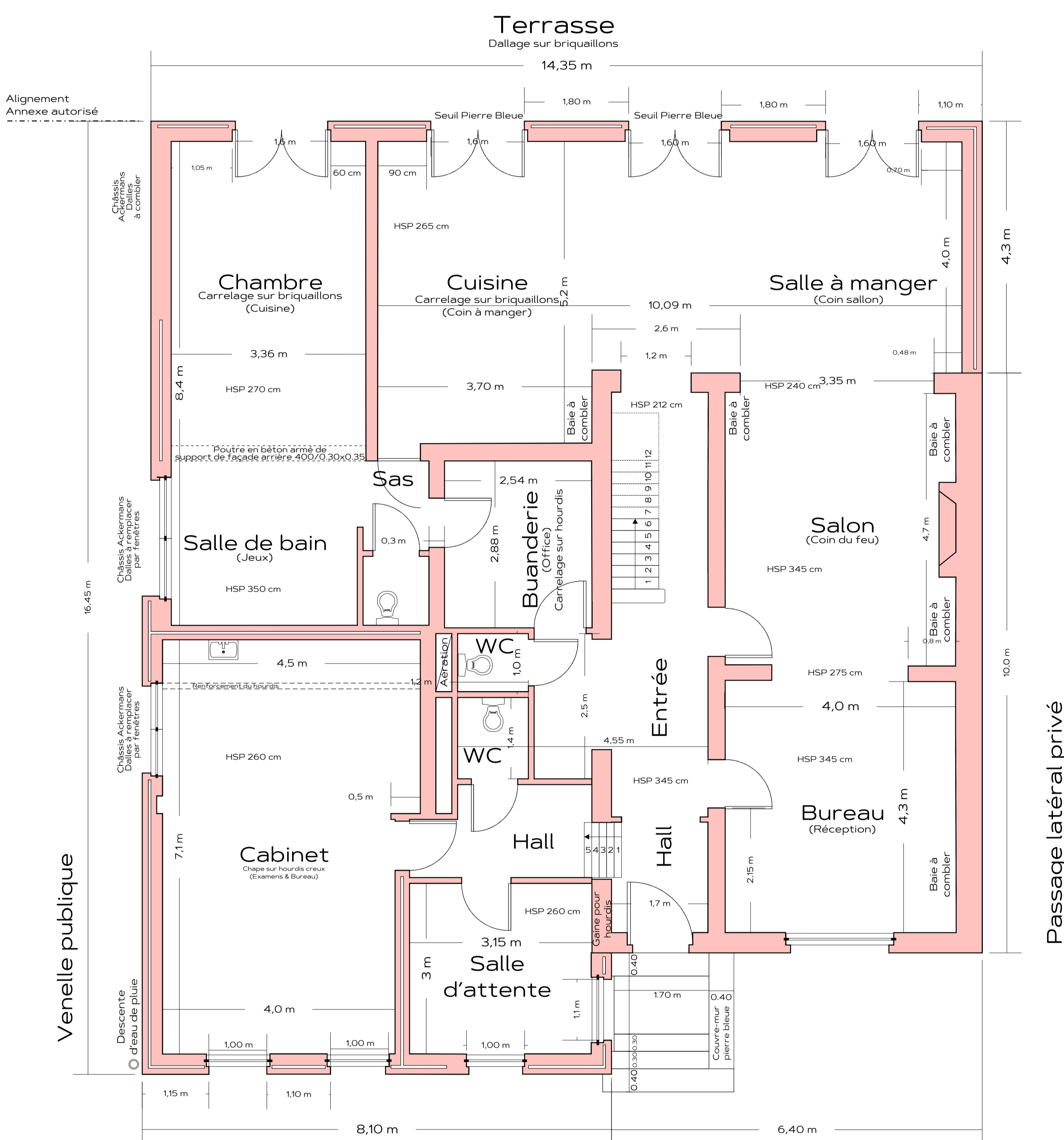
PLAN DU REZ DE CHAUSSEE
