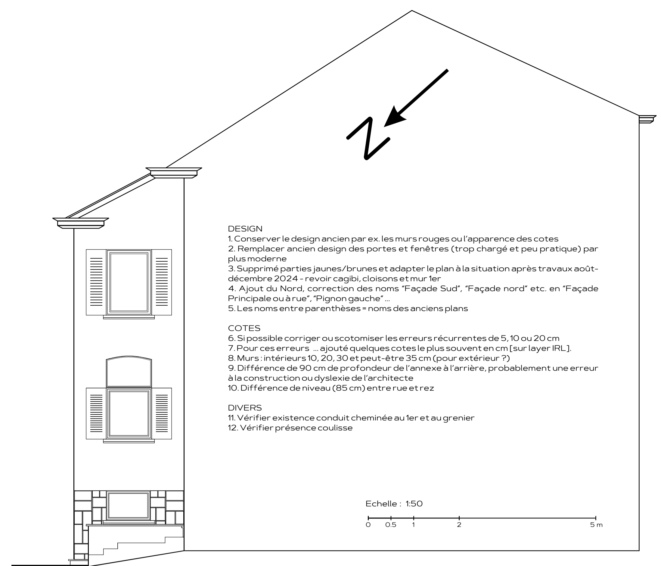
PIGNON DROIT Passage latéral privé
